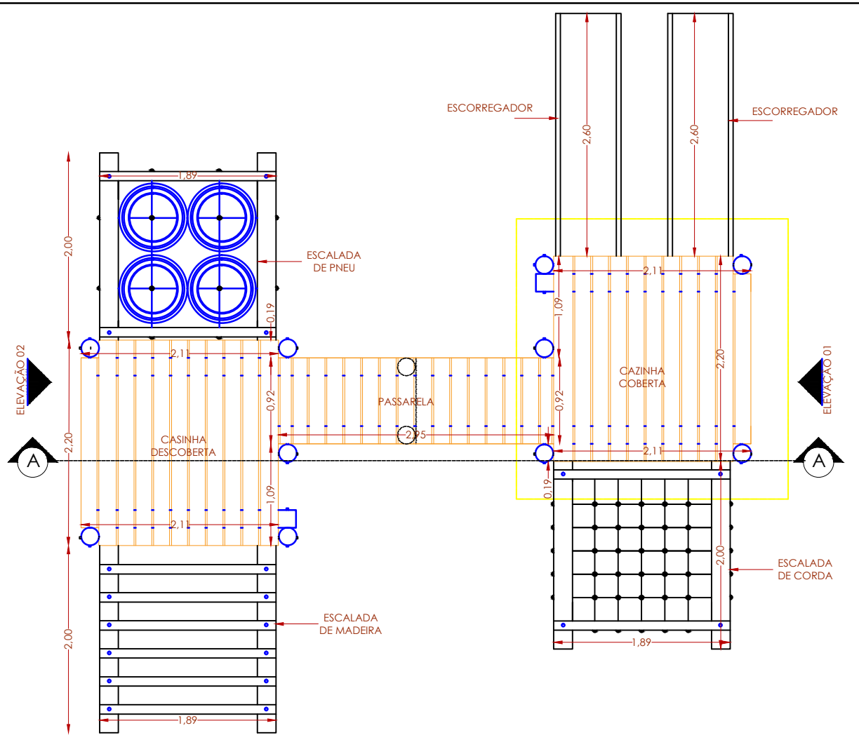
PLANTA BAIXA GERAL ESC:1:50
