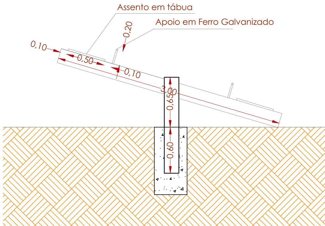
VISTA LATEAL ESC:1:50
