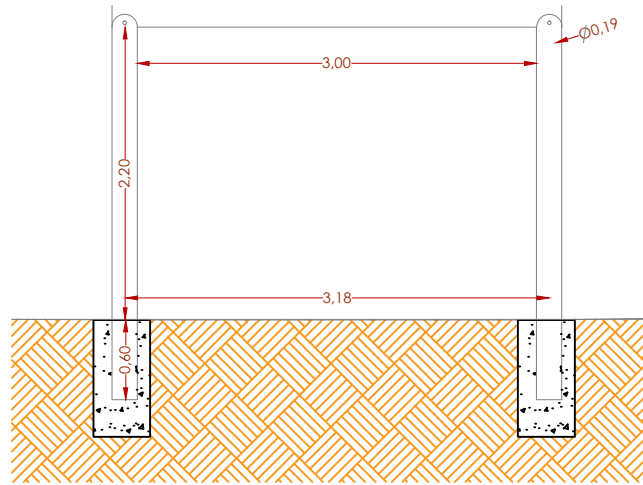
VISTA FRONTAL ESC:1:50
