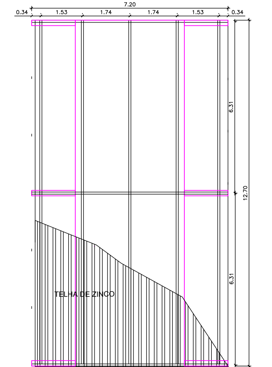
Planta de Cobertura 03 Esc: 1/75
