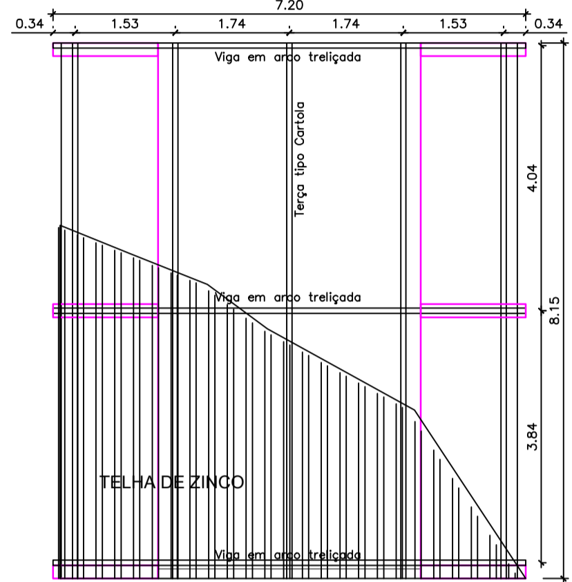
Planta de Cobertura 02 Esc: 1/75
