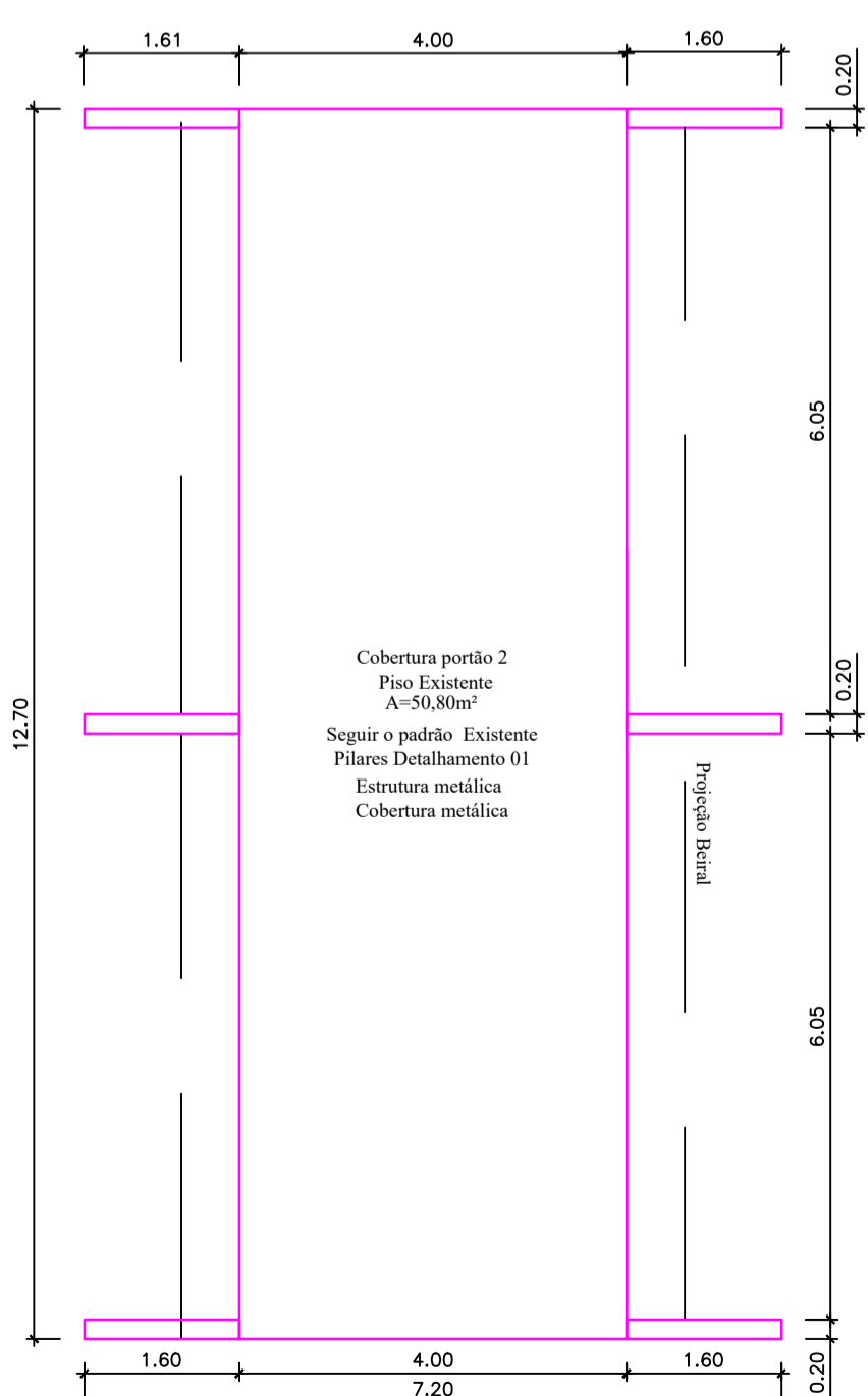
Planta Baixa Cobertura 03 Esc: 1/75
