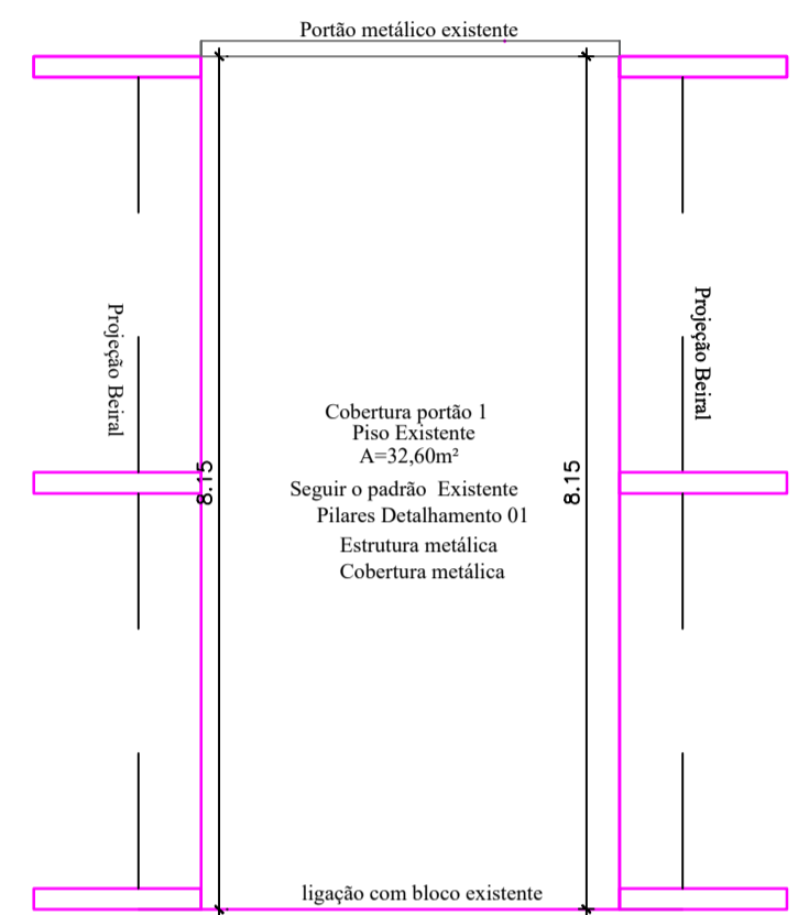
Planta Baixa Cobertura 02 Esc: 1/75
